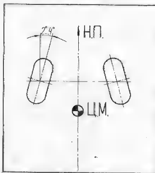
Рис.4. Схема развала колес в плаве
